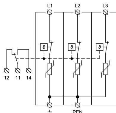
Vnútrotná schéma zapojenia
